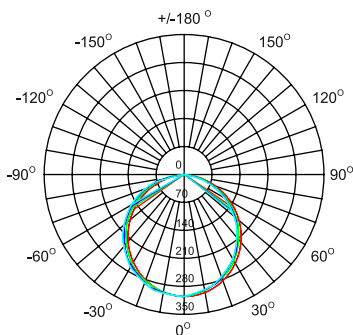
Diagrama fotometrica
