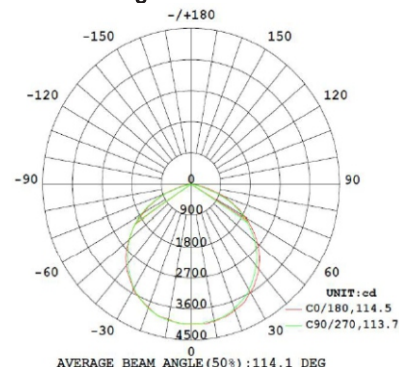
Diagrama fotometrica
