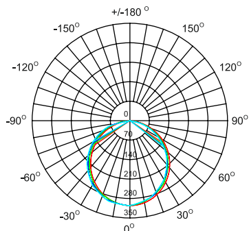
Diagrama fotometrica
